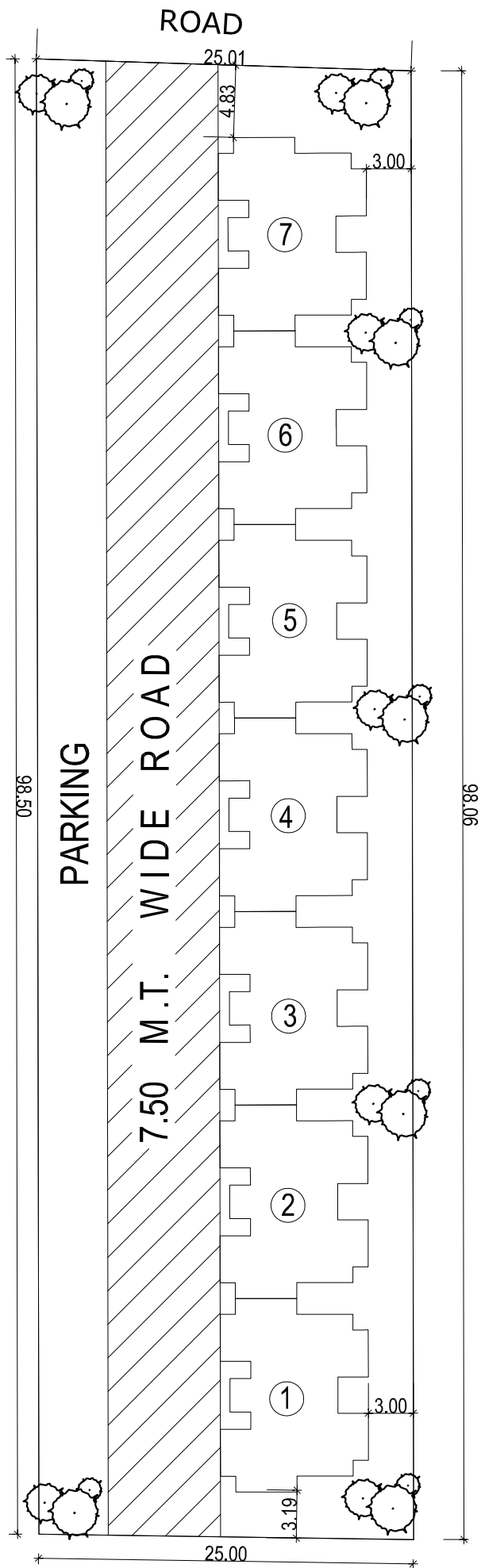
LAY-OUT OF AT T.P.NO-2,(UDHANA) F.P. NO.-94 PAIKI
